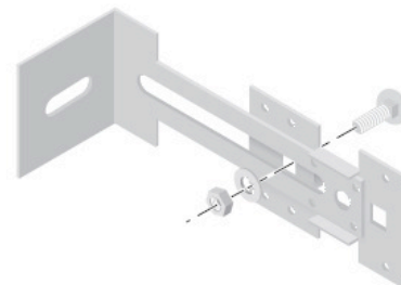
Equerelo L150 avec coulisse
