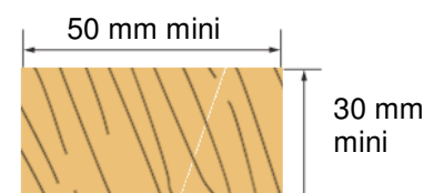
Pose directe sur le support
