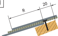
D - Pose à deux clous
