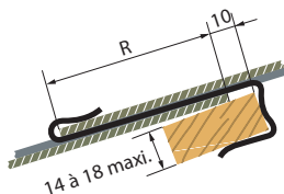
A - Crochet à pression pour lattage
