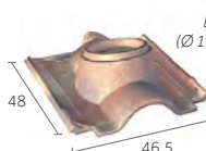
Tuile à douille (Ø int. : 150 mm)
