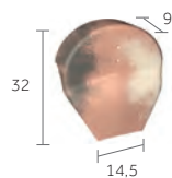
Fronton de rive ronde pour faîtière conique/demi-ronde de 40 (Petit modèle)
