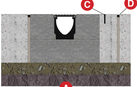
Pose en chaussée béton
