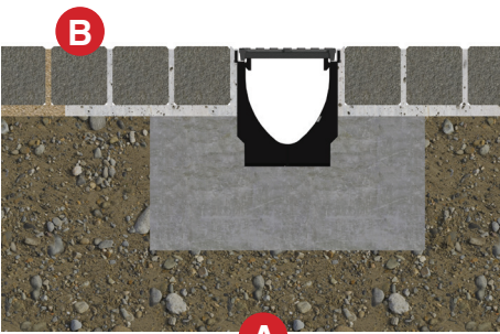
Pose en chaussée pavée
