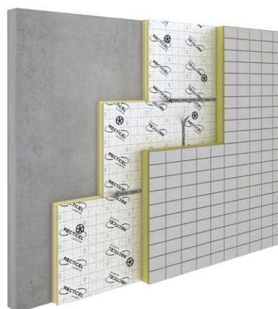
Exemple de pose de vêtiture
