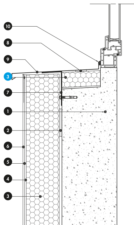
Fig. 23 : Coupe sur baies en service : appui maçonné trop court (coupe verticale) Cette solution ne peut être réalisée que si les drainages des feuilures ne sont pas occultés
