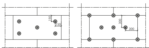
5 chevilles par panneau (soit 6,9 par m 2 )
