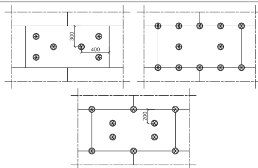
6 chevilles par panneau (soit 8,3 par m 2 )
