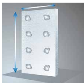
Fig. 1 : Exemple de répartition du mortier colle
