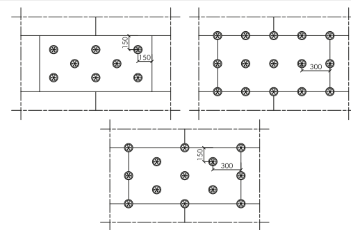
8 chevilles par panneau (soit 11.1 par m 2 )
