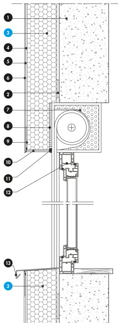
Fig. 26 : Coffre de volet roulant débordant du gros œuvre (coupe verticale)
