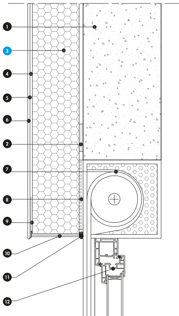
Fig. 25 : Coffre de volet roulant aligné au gros œuvre : fenêtre au nu intérieur (coupe verticale)
