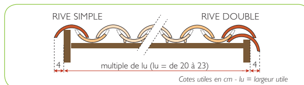
Cotes utiles en cm - lu = largeur utile
