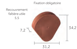
Fronton de rive à rabat pour faîtière demi-ronde
