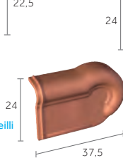
About de rive de 33 gauche
