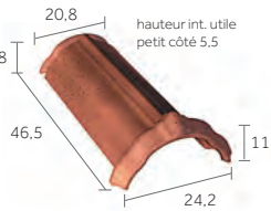
Arêtier de 40 à emboîtement
