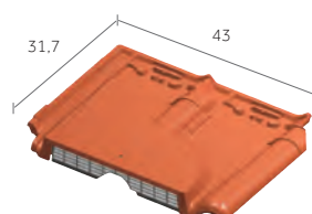
Tuile châtère grillagée (ouverture de 31 cm²)
