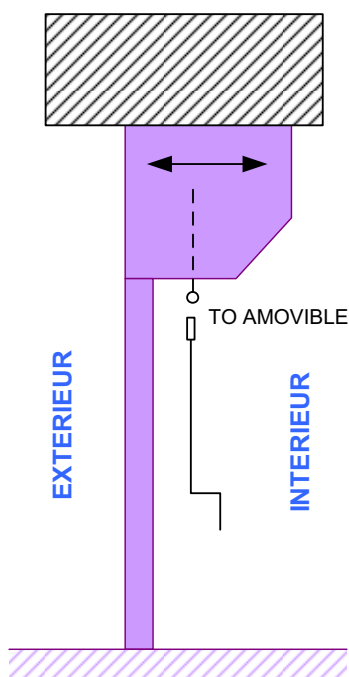
POSE SOUS DALLE
