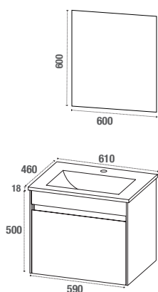
AGATE600CC AGATE600GP
