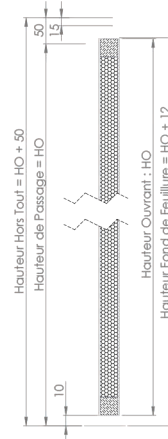
coupe verticale
