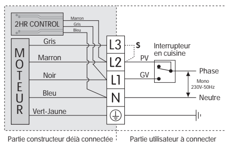
Schéma de câblage interrupteur va et vient
